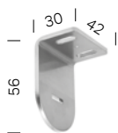
Universalträger aus Edelstahl (serienmäßig enthalten)
